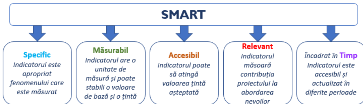
Figura 9: Indicatori SMART
